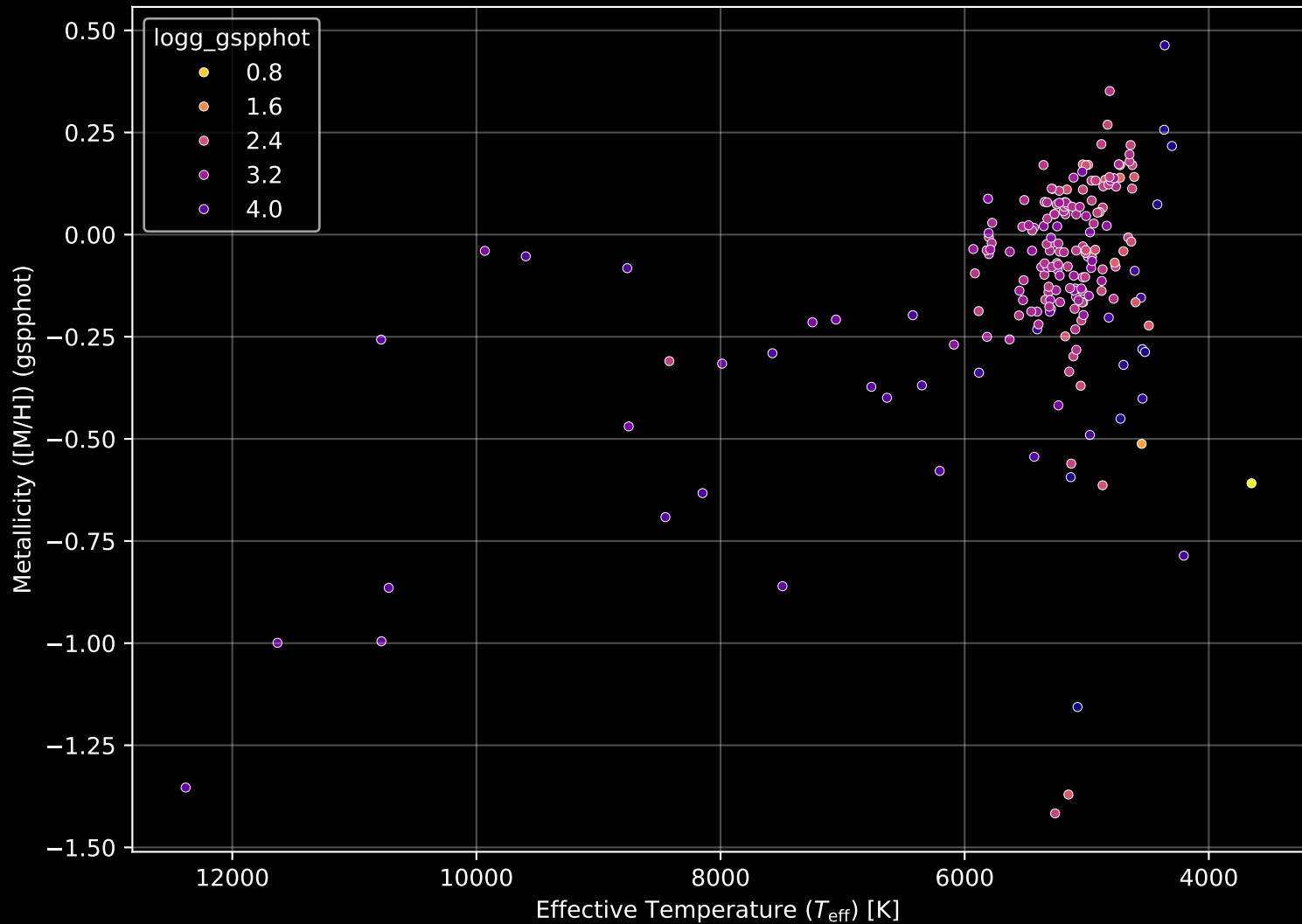
APOGEE DR17 Field: [173-12] Stellar Population Parameters (n= 203)
